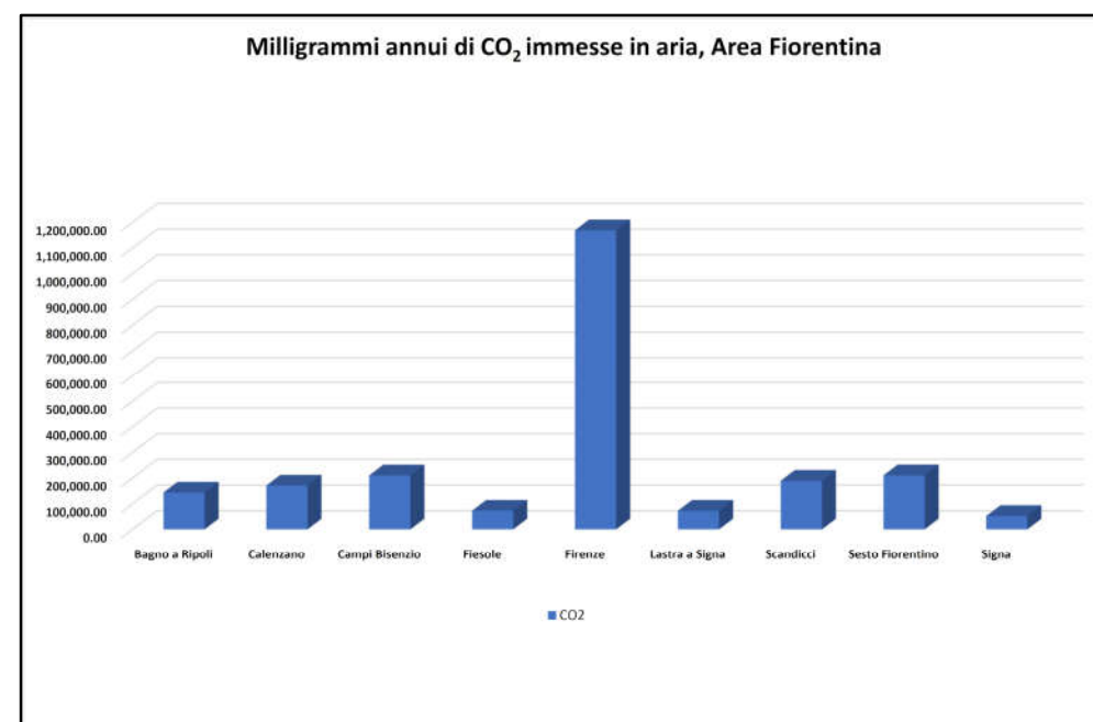
Figura 64 - Emissioni CO 2 Area Fiorentina. Fonte: IRSE, Regione Toscana
