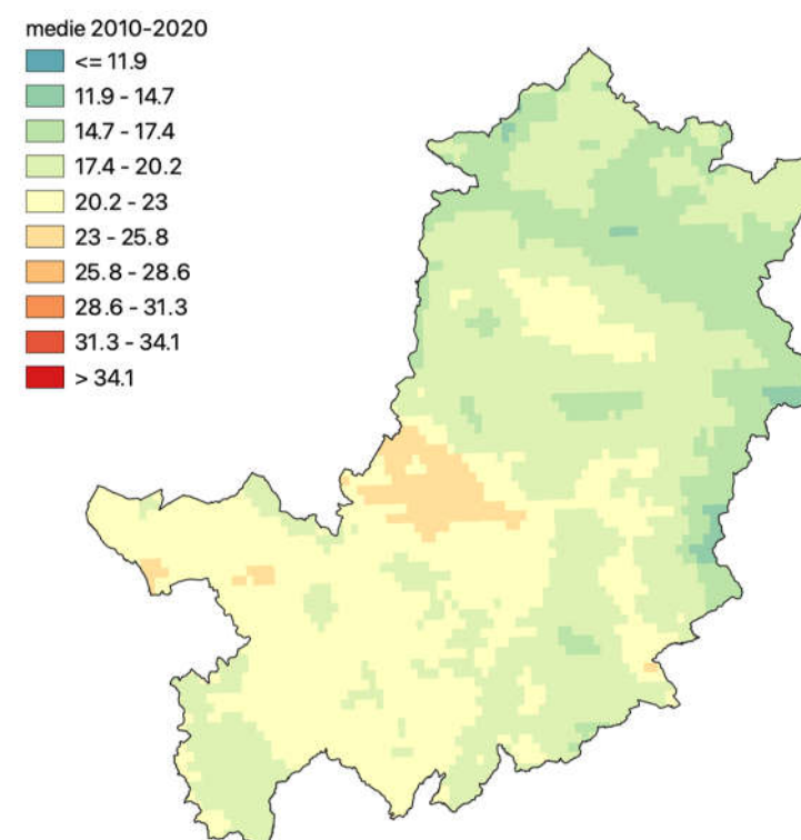
Figura 73 - Media delle temperature 2010-2019
