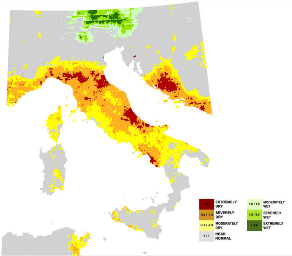
Figura 68 - SPI3 dell'Italia del 31-08-2017
