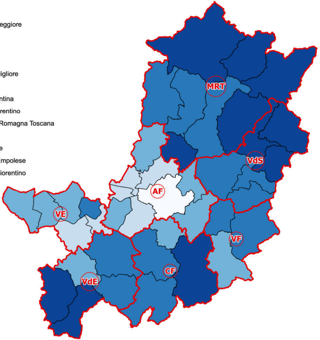
Figura 17 - Indicatore normalizzato a livello comunale
