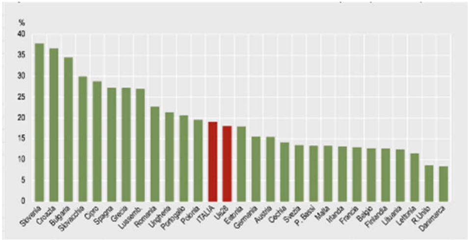
Figura 104 - la rete Natura2000 nei paesi dell'UE28 (2018)
