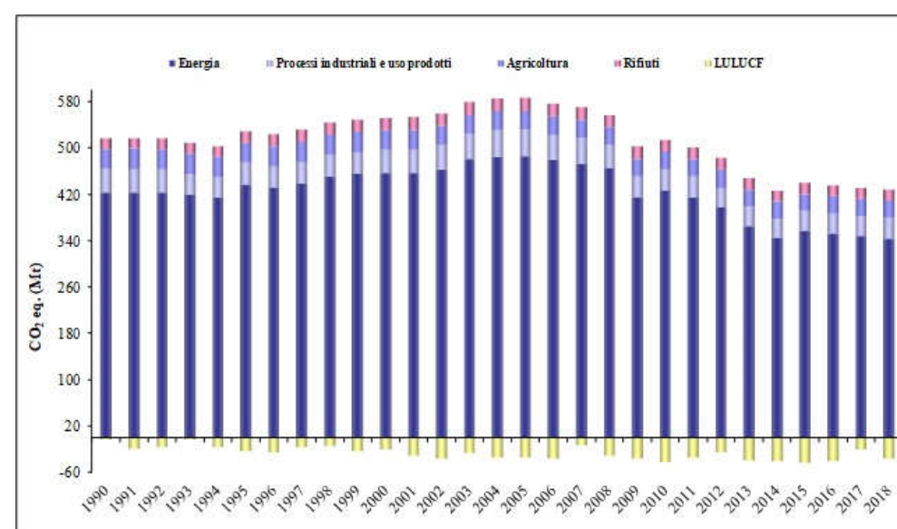
Figura 62 - Emissioni nazionali di gas climalteranti dal 1990 al 2018 per settore
