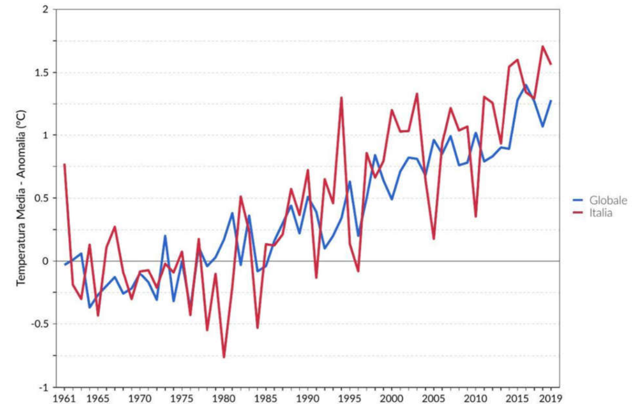
Figura 66 - Serie delle anomalie di temperatura media globale sulla terraferma e in Italia, rispetto ai valori climatologici normali
