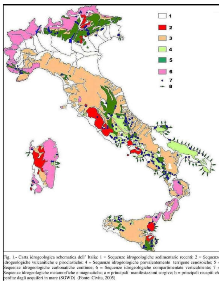
Figura 25 - Carta Idrogeologica dell'Italia. Fonte: Civita, 2005
