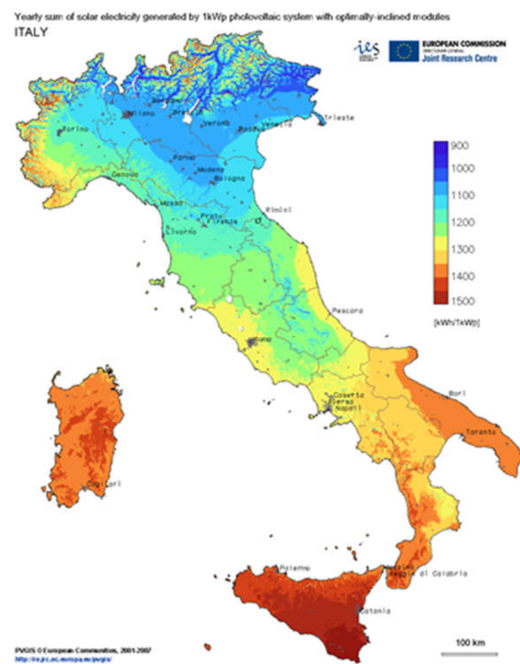
Figura 143 - Rendimento medio degli impianti fotovoltaici nel territorio italiano
