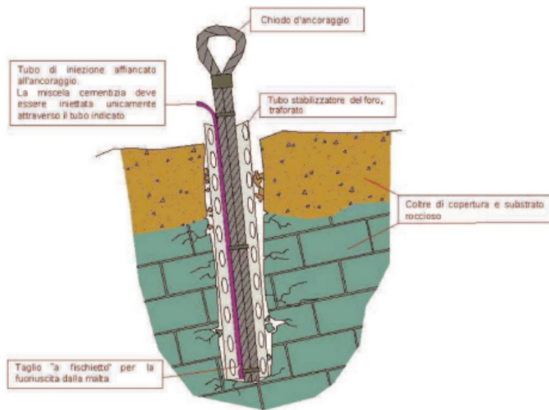
Sistema foro-chiodatura
