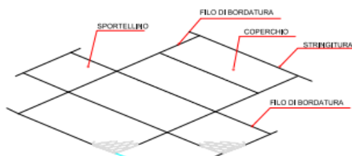
GABBIONE APERTO PER LA MESSA IN SCATOLA
